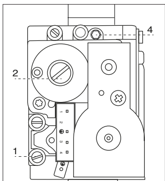
Plynový ventil 848 / Plynový ventil 848
