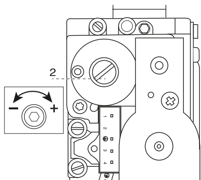
Plynový ventil 848 / Plynový ventil 848
