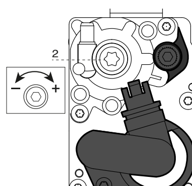
Plynový ventil 8205 / Plynový ventil 8205
