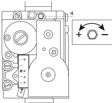
Plynový ventil 848 / Plynový ventil 848
